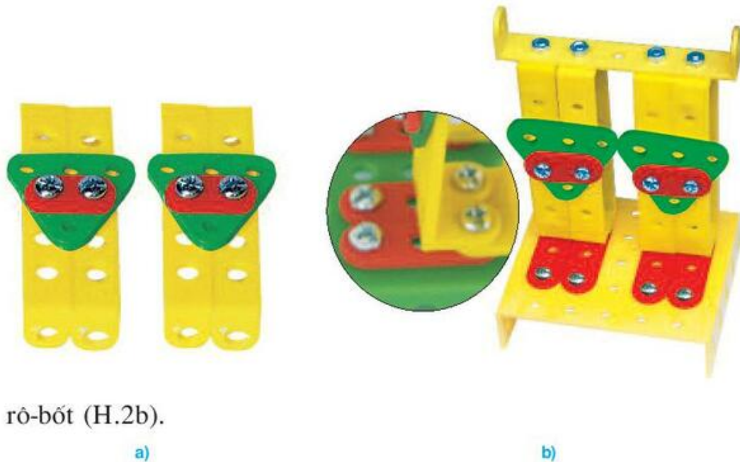
Hình 2. Lắp chân và thanh đỡ thân rô-bốt
